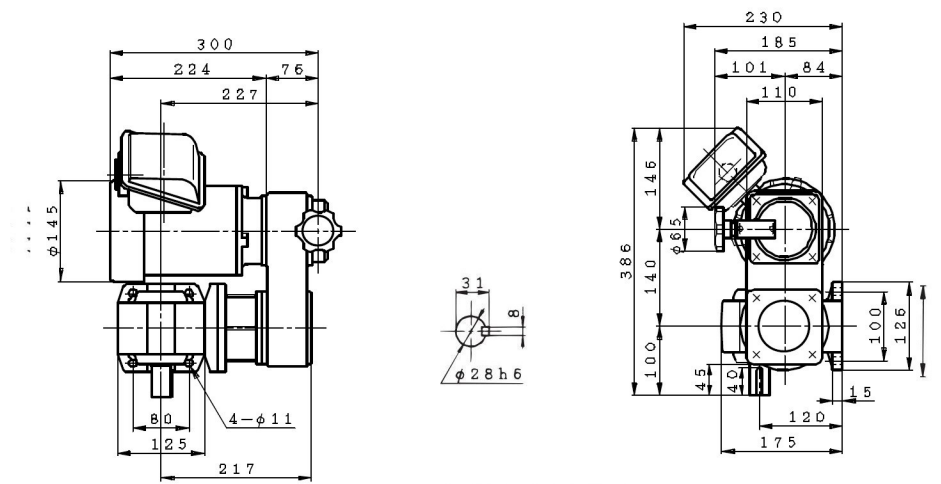
TH-4-5~60 (質量:22.4kg) (単位:mm)
