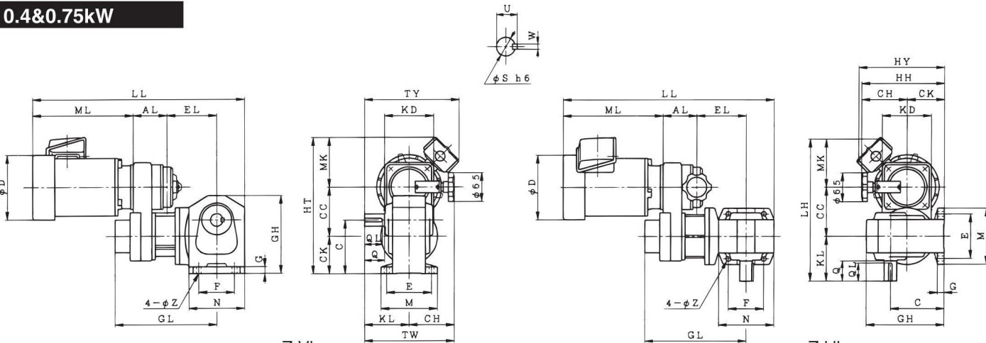
Z-VL Z-HL (単位:mm)
