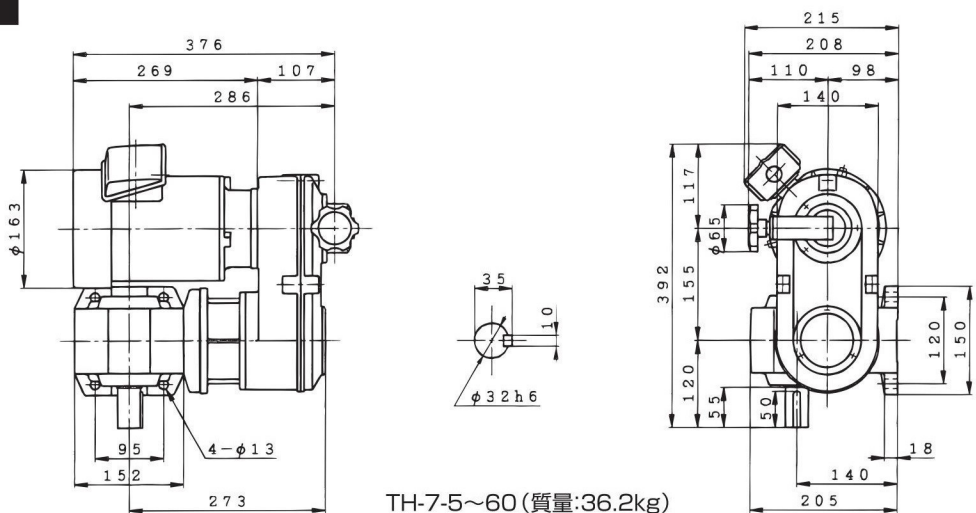
TH-7-5~60 (質量:36.2kg) (単位:mm)
