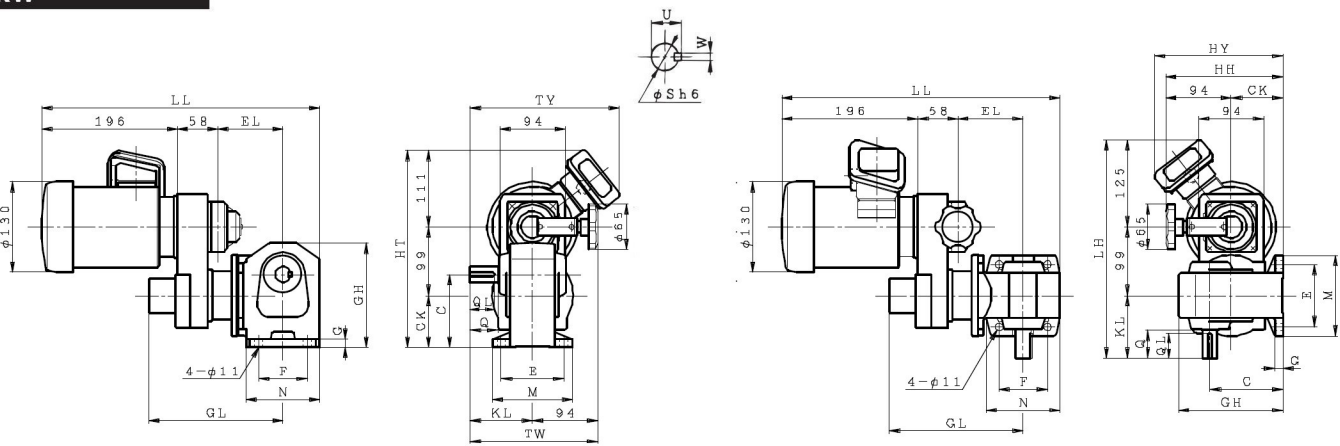
Z-VL Z-HL (単位:mm)
