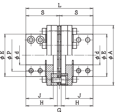
TCFFS-125B~200B 寸法図
