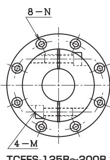
TCFFS-125B~200B 寸法図
