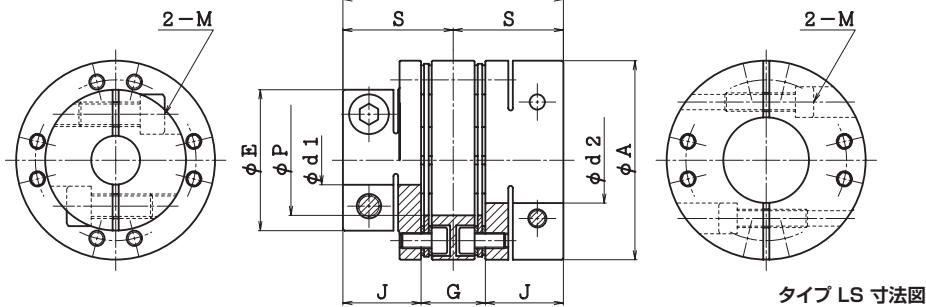
タイプ LS 寸法図
