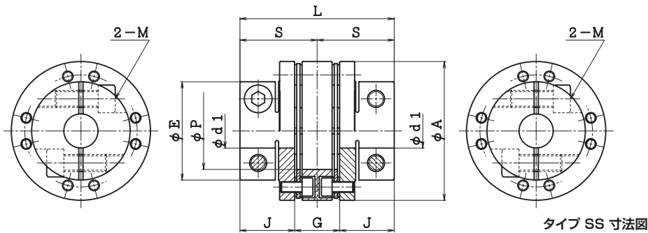
タイプ SS 寸法図
