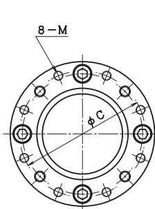
TCFFS-125~200 寸法図
